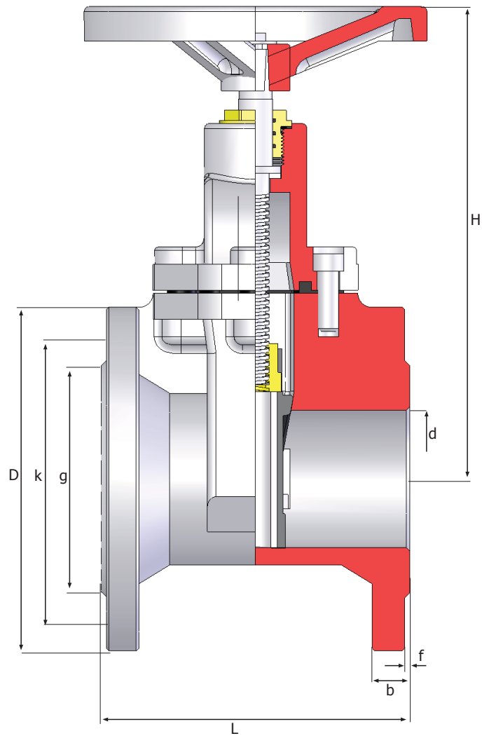
FAF 6000 PN16 ЗАДВИЖКА С ОБРЕЗИНЕННЫМ КЛИНОМ ИЗ ВЫСОКОПРОЧНОГО ЧУГУНА
