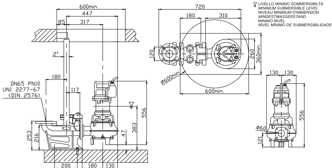
Dimensioni - Dimensions - Dimensions - Abmessungen - Dimensiones - Dimensões (mm)
